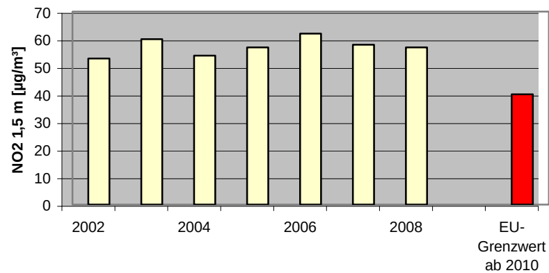
Kieler Straße Jahresmittelwerte NO 2
