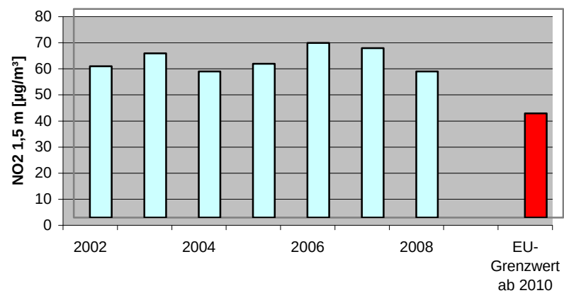
Stresemannstraße Jahresmittelwerte NO 2
