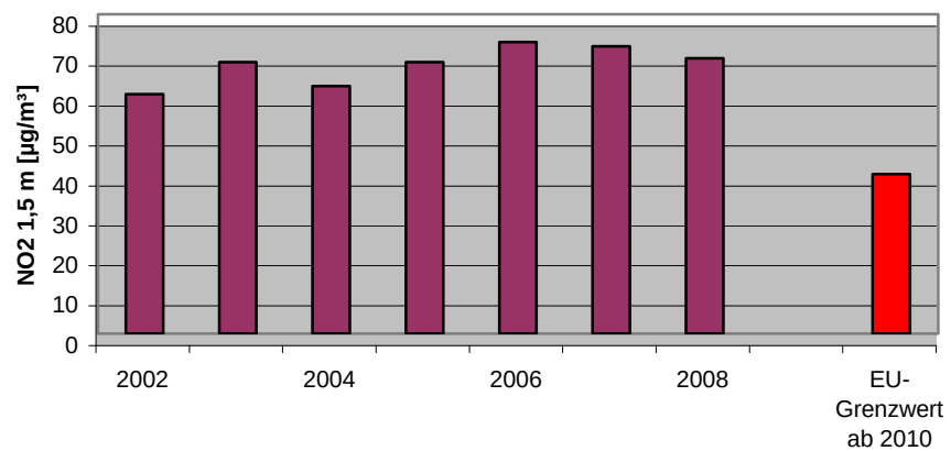
Max-Brauer-Allee Jahresmittelwerte NO 2
