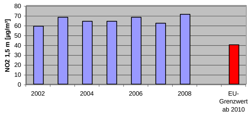
Habichtstraße Jahresmittelwerte NO 2
